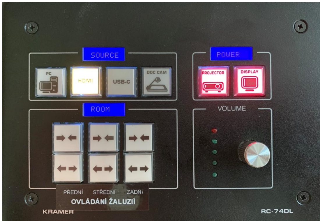
Obrázek 1: ovládací panel
